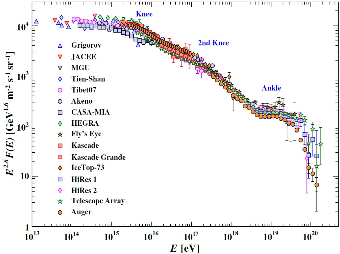
Figura 1.1: Espectro de energ3a de rayos c3smicos obtenido a partir de los datos de los detectores m3s importantes en los rangos de energ3a 10^{13} \text{ eV} < E < 5 \times 10^{20} \text{ eV} . Se observa como cambia el flujo comparado con E^{2.6} y se pueden ver las caracter3sticas morfol3gicas m3s relevantes, la 'rodilla', la 'segunda rodilla', el 'tobillo' y la supresi3n de espectro a muy altas energ3as. Obtenido de [8].
